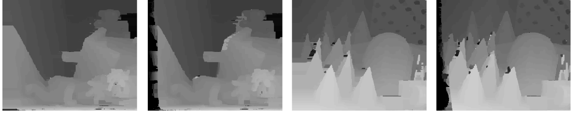
Abbildung 31: Die Verdeckungsbehandlung benötigt 55 Prozent der gesamten Laufzeit, verbessert dafür die Ergebnisse deutlich. Die linken Bilder der beiden Stereobildpaare zeigen jeweils die Resultate mit Verdeckungsbehandlung. Bei den rechten Bildern wurde die Verdeckungsbehandlung weggelassen.
