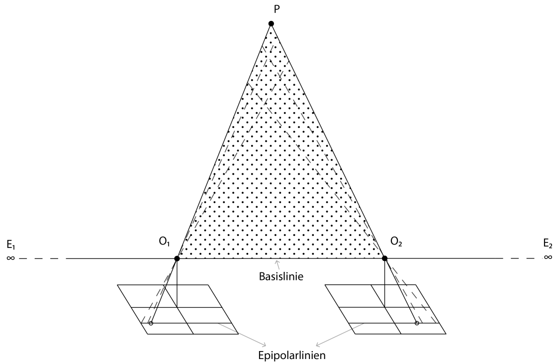
Abbildung 4: Bei der achsenparallelen Kameraanordnung decken sich die Epipolarlinien mit den Zeilen der Bilder. Daher entfällt eine Bestimmung der Epipolarlinien. Der korrespondierende Bildpunkt eines Szenepunktes P liegt nun immer auf der korrespondierenden Zeile im anderen Bild. Durch die Begradigung wandern die Epipole E_1 und E_2 ins Unendliche, weil sich die Epipolarlinien nicht mehr schneiden. O_1 und O_2 sind die Projektionszentren der Kameras. Quelle: Vorlage aus [29].
