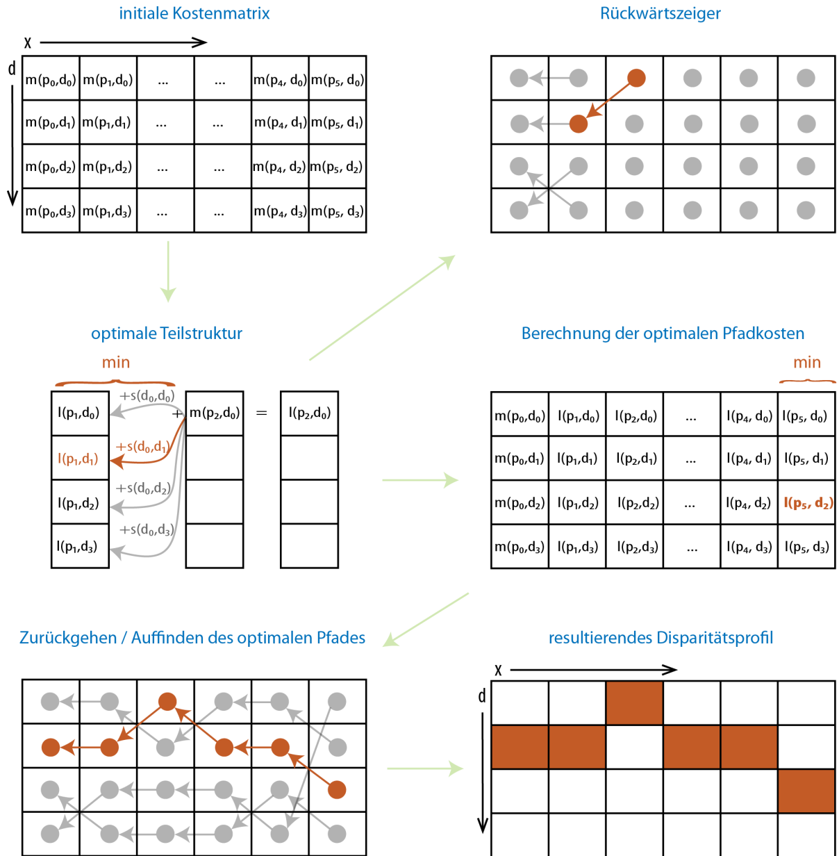
Abbildung 13: Die einzelnen Schritte zur Berechnung von Disparitäten durch Energieminimierung via dynamische Programmierung entlang von Bildzeilen. Das sukzessive optimale Lösen von Teilproblemen führt zu einer globalen optimalen Lösung.
