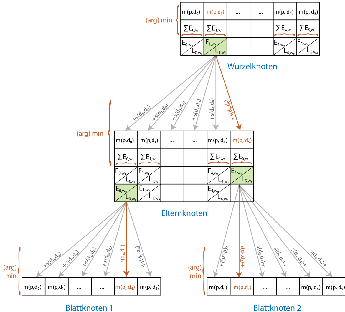
Abbildung 16: Die Bestimmung der optimalen Disparität für den Wurzelknoten mithilfe dynamischer Programmierung angewendet auf einen Baum. Die Vorgehensweise ähnelt der Vorgehensweise von dynamischer Programmierung entlang von Zeilen.
