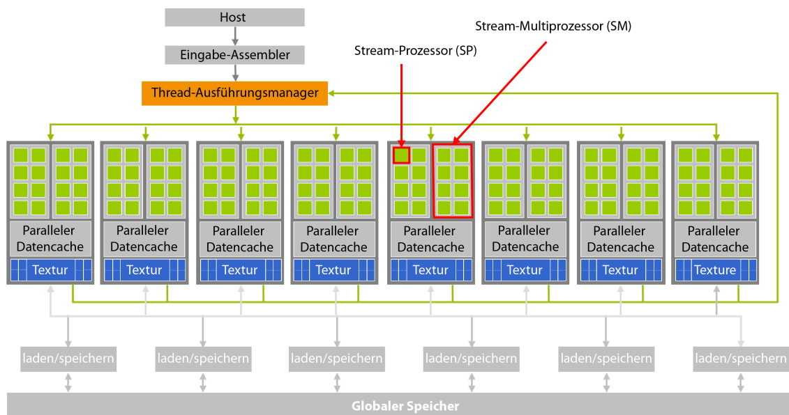
Abbildung 22: Aufbau des G80-Graphikprozessors als Beispiel für eine CUDA-fähige Architektur. Quelle: [116].
