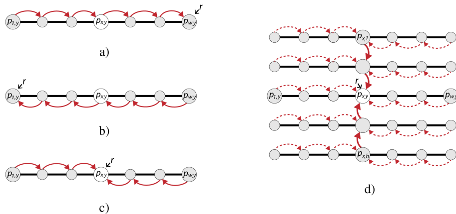
Abbildung 19: a) Vorwärtsdurchlauf mit dynamischer Programmierung in horizontaler Richtung b) Rückwärtsdurchlauf c) Durch die Kombination von Vorwärts- und Rückwärtsdurchlauf lassen sich jene Kosten ermitteln, welche die optimalen Kosten von linker und rechter Seite kommend darstellen. d) zeigt die Berechnung der minimalen Kosten eines horizontalen Baumes, wurzelnd im Pixel p_{x,y} . Dazu optimiert man in vertikaler Richtung unter Verwendung der Werte aus der horizontalen Optimierung.
