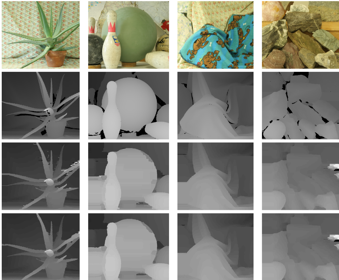
Abbildung 35: Die Ergebnisse der GPU-Implementierung für die Stereobildpaare Aloe, Bowling2, Cloth3 und Rocks2 des Middlebury-Datensatzes 2006. Die erste Reihe (von oben) zeigt die Referenzbilder, die zweite die tatsächlichen Disparitäten, die dritte die Disparitätskarten der GPU-Implementierung ohne bilateraler Medianfilterung und die letzte die Disparitätskarten nach der Filterung.
