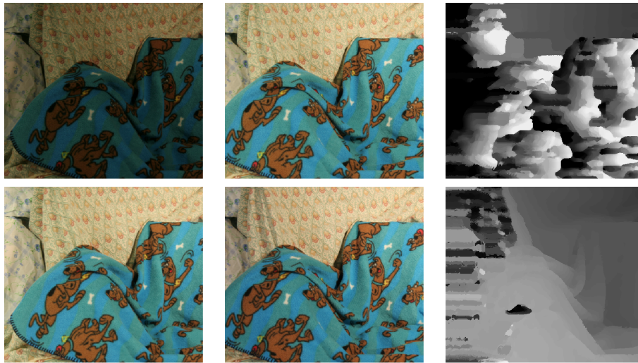
Abbildung 36: Radiometrische Unterschiede im linken und rechten Bild können von der hier eingesetzten Metrik kaum kompensiert werden. Die Ergebnisse verschlechtern sich signifikant. Die erste Reihe zeigt linkes und rechtes Bild des Bildpaars Cloth3 aufgenommen mit verschiedenen Belichtungszeiten und die damit berechnete Disparitätskarte. Die zweite Reihe zeigt linkes und rechtes Bild bei einer unterschiedlichen Beleuchtung (mit gleichen Belichtungszeiten) und die berechnete Disparitätskarte.
