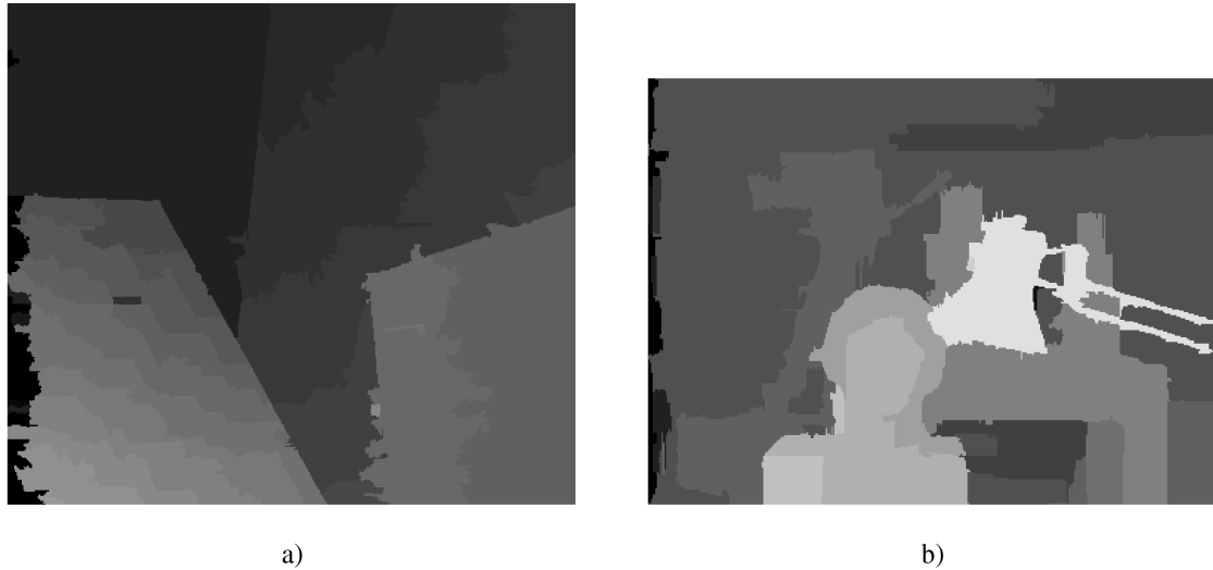
Abbildung 17: Ergebnisse der Disparitätsoptimierung via dynamische Programmierung auf einem Baum, wie in [105] beschrieben, für das Stereobildpaar a) Venus und b) Tsukuba. Vergleicht man die Resultate mit den Resultaten dynamischer Programmierung entlang von Zeilen (Abb. 12), zeigt sich, dass keine Streifenbildung mehr auftritt und die Ergebnisse im Allgemeinen besser ausfallen. Quelle: [51].
