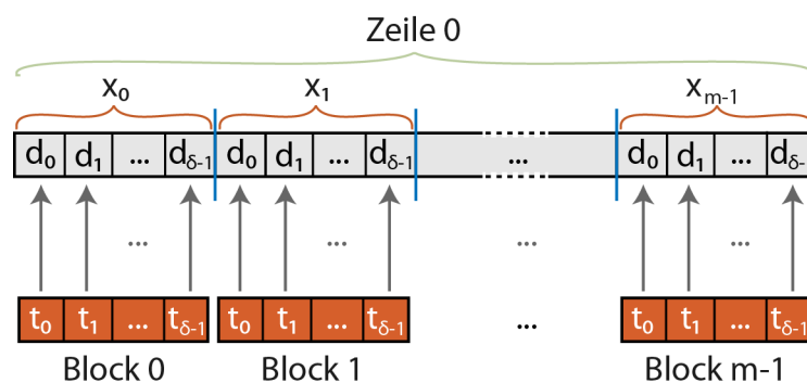
Abbildung 25: Bei den Durchläufen dynamischer Programmierung liest je ein Block gut koordiniert alle Disparitätskosten für ein Pixel. Dafür besitzt jeder Block so viel Threads, wie es Disparitätsstufen gibt. So schafft man es, die hohe Bandbreite zum globalen Speicher effizient zu nutzen.
