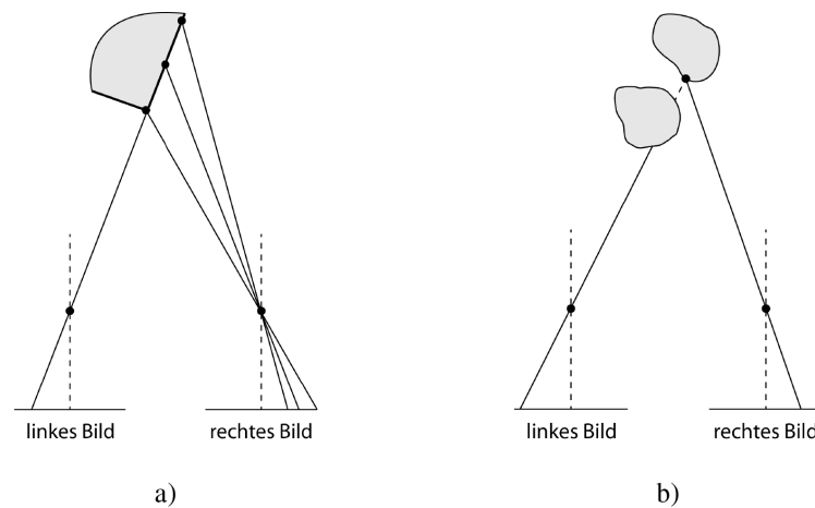
Abbildung 6: a) Wenn mehrere Szenepunkte auf dem Sichtstrahl einer Kamera liegen, wird die Eindeutigkeitsbedingung verletzt. b) Bei Verdeckungen kommt es ebenfalls zu einer Verletzung der Bedingung, da manche Pixel nur in einem Bild auftauchen. Quelle: [45].
