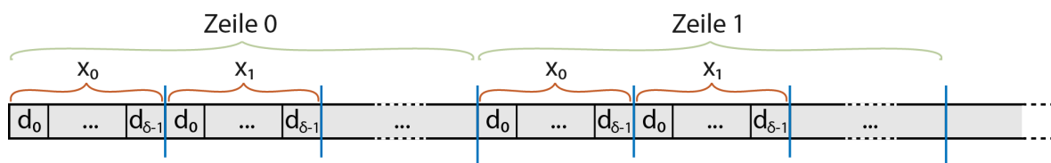
Abbildung 24: Organisation des DRV's. Die gewählte Anordnung erlaubt ein effizientes Lesen der Werte aus dem globalen Speicher zu einem späteren Zeitpunkt. Die Disparitätsstufen gehen von d_0 ... d_{\delta-1} mit \delta als Anzahl der möglichen Disparitätsstufen.
