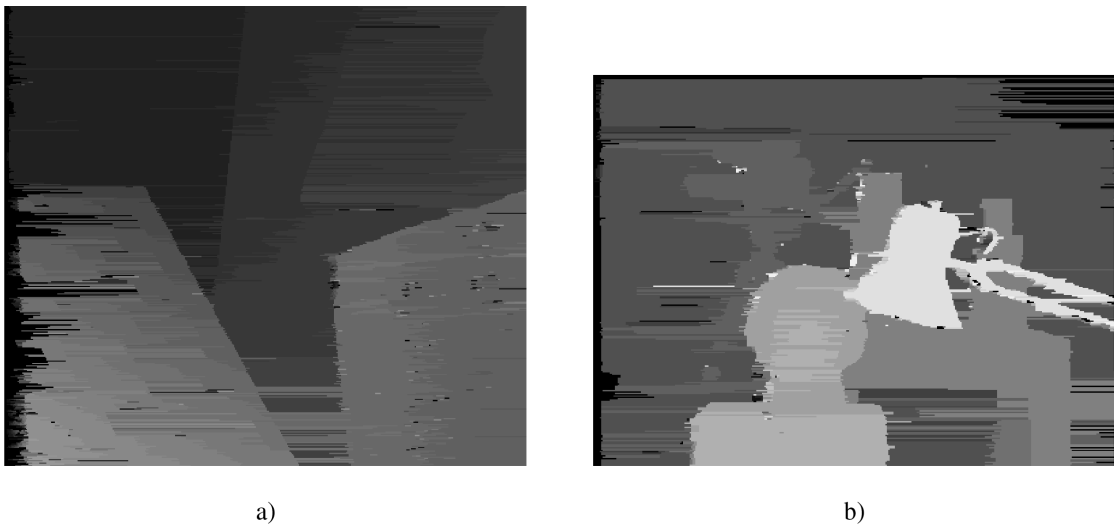
Abbildung 12: Ergebnisse der Bildzeilenoptimierung mit dynamischer Programmierung für die Stereobildpaare a) Venus und b) Tsukuba. Weil die Zeilen unabhängig voneinander optimiert werden, besteht keine Konsistenz über unterschiedliche Bildzeilen hinweg. Dieser Umstand führt zu der deutlich sichtbaren Streifenbildung in den berechneten Disparitätskarten. Quelle: [51].
