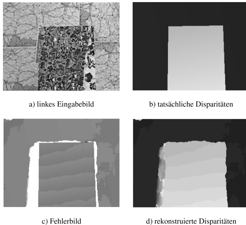
Abbildung 8: Bei Fenstermethoden mit starrem Fenster kommt es in der Nähe von Disparitätsdiskontinuitäten zu einer Verdickung des Vordergrundes. In diesen Regionen befinden sich mehrere Disparitätspopulationen innerhalb desselben Fensters, und weil der Vordergrund häufig stärker texturiert ist als der Hintergrund, setzt sich in der Regel die Disparitätspopulation des Vordergrundes durch. Zur Berechnung der Disparitäten setzte man ein starres 21x21 Fenster ein und nutzte die SAD als Ähnlichkeitsmaß. Quelle: [41].
