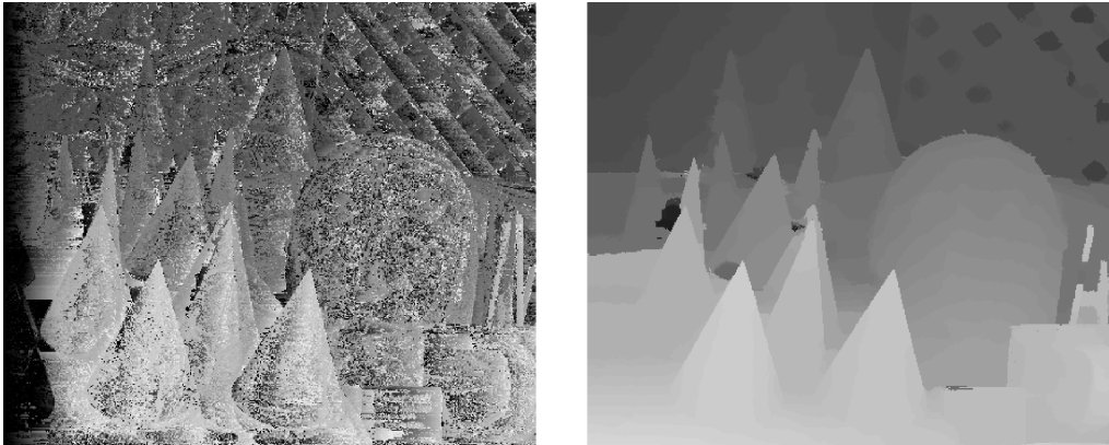
Abbildung 37: Die Wirkung der eingesetzten Optimierung veranschaulicht anhand des Stereobildpaares Cones. Links die Disparitätskarte vor der Optimierung und rechts die Disparitätskarte nach der Optimierung.
