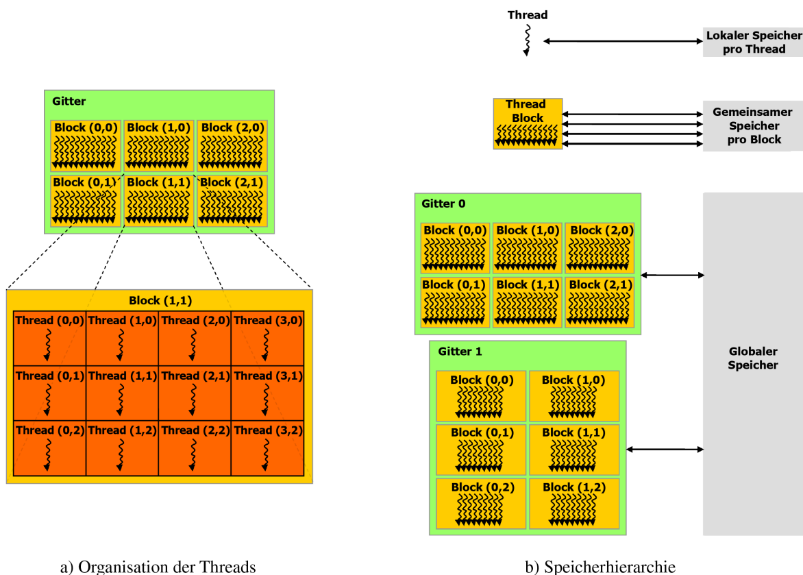
Abbildung 23: Zwei wichtige Komponenten des Programmiermodells von CUDA: a) die Organisation der Threads und b) die Speicherhierarchie. Quelle: [113].
