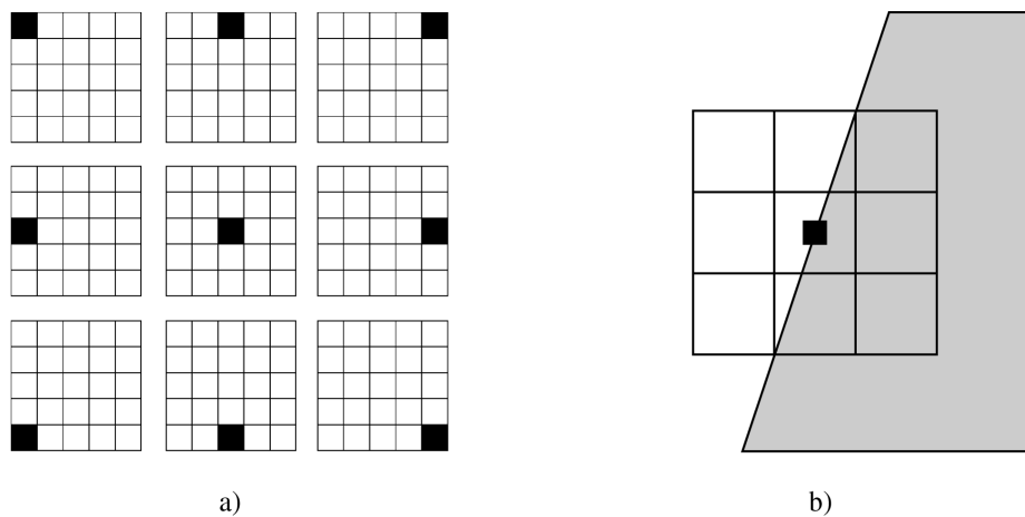
Abbildung 10: Der Sinn von variablen oder multiplen Fenstern ist, dass lediglich jener Bereich zur Bestimmung der Ähnlichkeit eingesetzt wird, welcher die Disparitätspopulation des Pixels von Interesse enthält. a) In [61] gebraucht man neun in ihrer Position leicht verschobene Fenster und selektiert das Fenster, welches die niedrigsten Kosten verursacht. b) In [64] unterteilen Hirschmüller et al. einen Bereich um das zentrale Pixel in neun Sektoren. Zur Korrelation werden die vier besten und der mittlere Sektor eingesetzt. Quellen: a) [61] b) [64].
