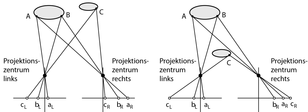
Abbildung 7: Kleine Objekte im Vordergrund bewirken eine Verletzung der Reihenfolgebedingung. Links besitzen die Objekte annähernd denselben Abstand von den Bildebenen. Die Projektionen der Punkte treffen in der Reihenfolge c , b , a auf die Bildebenen. Rechts befinden sich die Objekte unterschiedlich weit von den Ebenen entfernt. Auf die rechte Bildebene treffen die Projektionen der Punkte nun in der veränderten Reihenfolge b_R , a_R , c_R auf. Quelle: [2][46].
