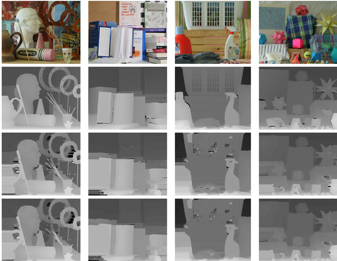
Abbildung 34: Die Ergebnisse der GPU-Implementierung für die Stereobildpaare Art, Books, Laundry und Moebius des Middlebury-Datensatzes 2005. Die erste Reihe (von oben) zeigt die Referenzbilder, die zweite die tatsächlichen Disparitäten, die dritte die Disparitätskarten der GPU-Implementierung ohne bilateraler Medianfilterung und die letzte die Disparitätskarten nach der Filterung.
