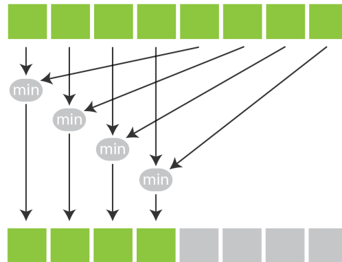
Abbildung 26: Grundgedanke der parallelen Reduktion. Quelle: [110].
