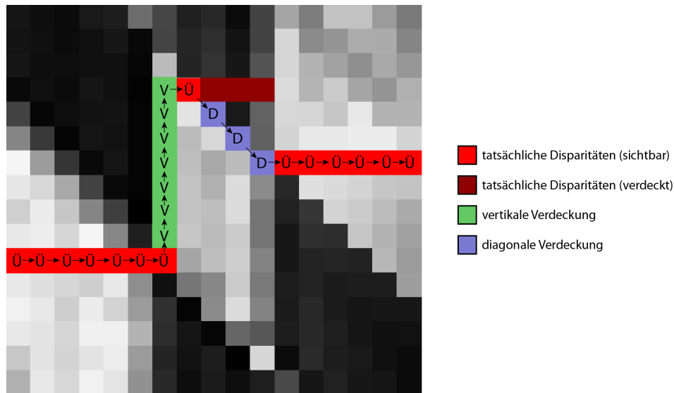
Abbildung 14: Forcierung der Reihenfolgebedingung nach [61]. Zu sehen ist ein Ausschnitt des DRBs aus Abbildung 11 d). Wählt man die Verdeckungskosten für vertikale und diagonale Sprünge zu hoch, findet man mit dynamischer Programmierung nicht den korrekten Pfad, weil ein Pfad mit falschen Korrespondenzen womöglich billiger ist. In der Abbildung würde der Pfad dann nicht zum einzelnen übereinstimmenden Pixel nach oben springen, sondern einen direkteren Weg zwischen den beiden Übereinstimmungssequenzen links und rechts ausmachen.
