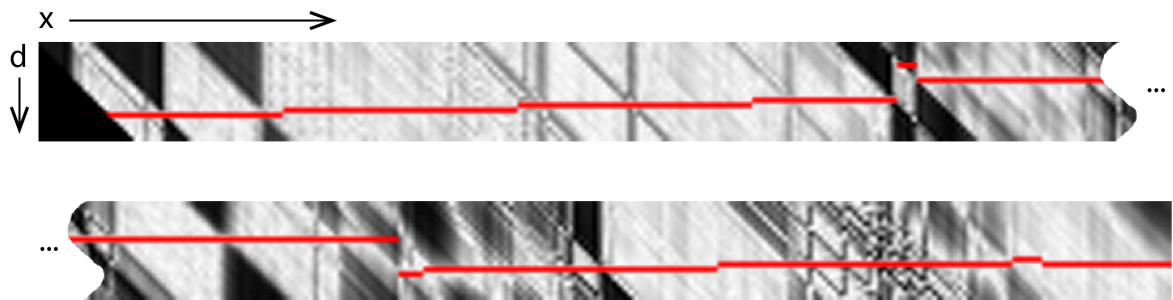
d) DRB für Zeile 250 des Stereobildpaares Venus (tatsächliche Disparitäten rot markiert)
