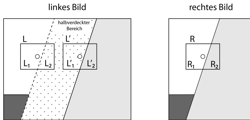
Abbildung 9: In der Nähe von Diskontinuitäten mit halb verdeckten Regionen tritt ein Entscheidungskonflikt auf. Welche Fenster übereinstimmen, hängt von der Beschaffenheit der halb verdeckten Region ab. Quelle: [55].
