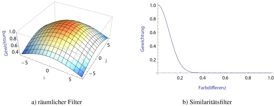
Abbildung 27: Die gaußschen Funktionen für den bilateralen Medianfilter. Beim Similaritätsfilter wird die Farbdifferenz zwischen zwei RGB-Farben auf normalisierten Farbkanäle zwischen 0 und 1 ermittelt, deshalb die niedrigen Werte.
