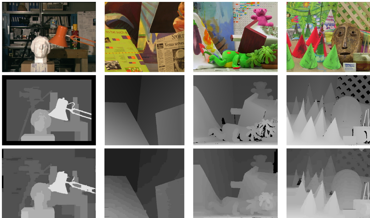
Abbildung 20: Die linken Bilder (oberste Reihe), die tatsächlichen Disparitäten (mittlere Reihe) und die nach [9] berechneten Disparitätskarten (unterste Reihe) der Stereobildpaare Tsukuba, Venus, Teddy und Cones des Middlebury-Datenbestandes. Die berechneten Disparitätskarten weisen einen glatten Verlauf innerhalb von Objekten auf und auch die Ränder von Objekten werden korrekt wiedergegeben. Trotz Glattheitsbedingung bleiben kleinere Details erhalten. Quellen: [9][51].
