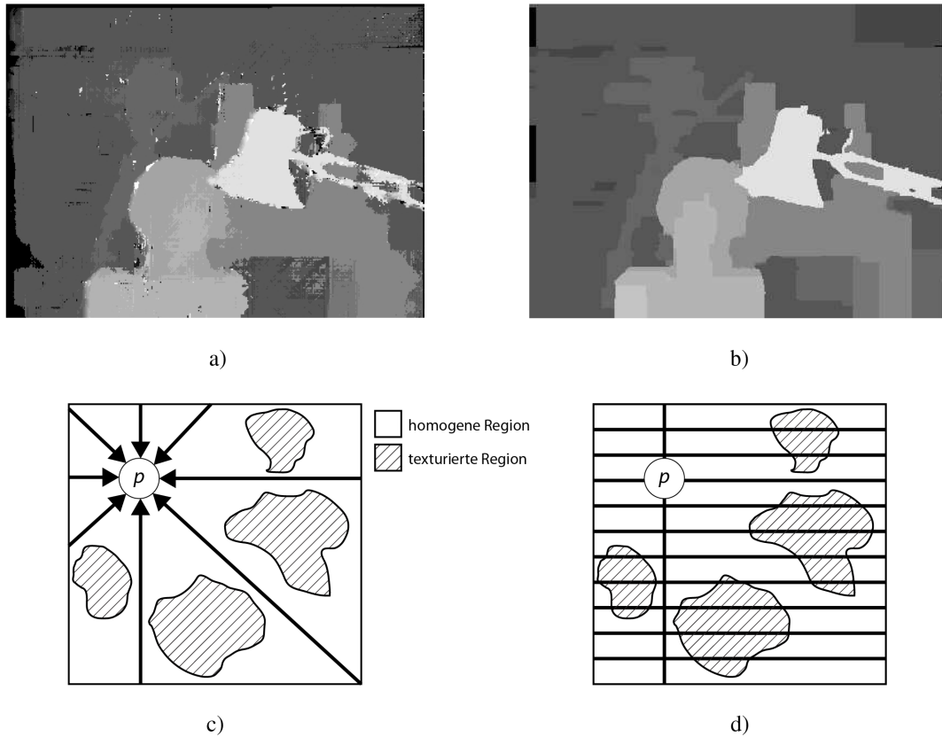
Abbildung 21: a) Disparitätskarte des Stereobildpaares Tsukuba berechnet mit einer Reimplementierung von [103] b) Disparitätskarte nach [9]. In a) tauchen vermehrt isolierte Pixel auf, die entstehen, wenn die Aggregationspfade bei den Durchgängen dynamischer Programmierung nicht ausreichend Textur enthalten (c)). In b) tritt dieses Problem nicht auf, weil jeder Baum, der zur Aggregation eingesetzt wird, alle Pixel des Referenzbildes enthält (d)). Quellen: a), c) und d) [109] b)[9].
