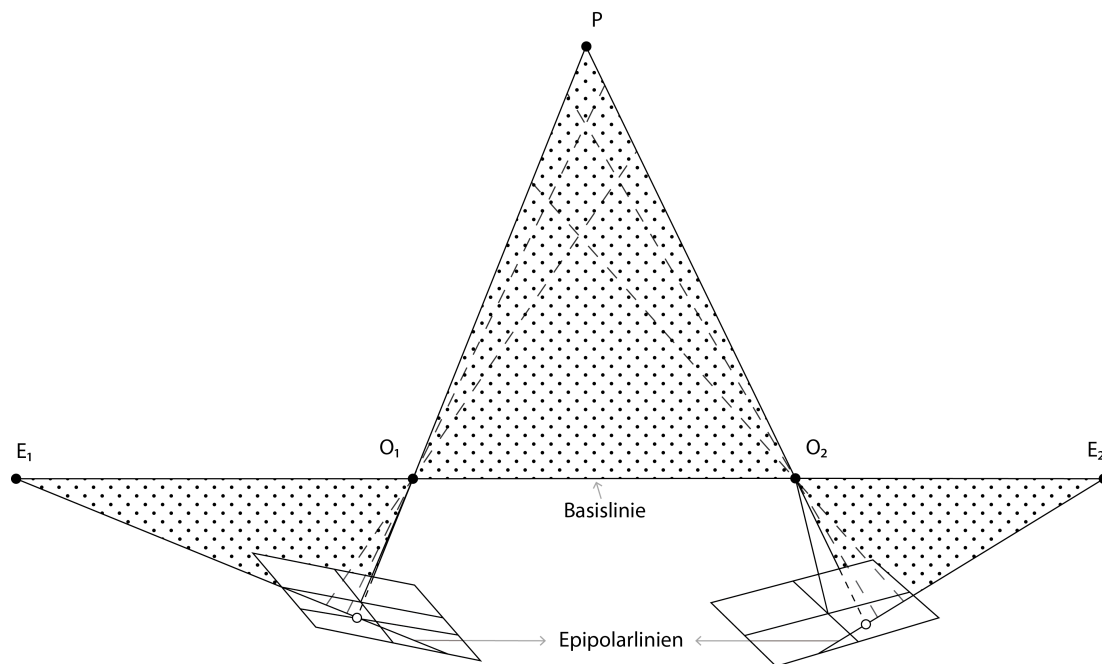
Abbildung 3: Bei der konvergenten Kameraanordnung verlaufen die Epipolarlinien quer durch die Bildfläche der Kamera. Die Epipolarlinien ergeben sich aus der Schnittfläche der Epipolarebene mit den Bildebenen der Kameras. Die Epipolarebene wird durch die zwei Projektionszentren der Kameras O_1 und O_2 , sowie einem Szenepunkt P definiert. Alle Epipolarlinien einer Bildebene schneiden sich im Epipol. E_1 und E_2 beschreiben je den Epipol für die Bildebene der linken und rechten Kamera. Der korrespondierende Bildpunkt eines Szenepunktes P liegt immer auf der dazugehörigen Epipolarlinie im anderen Bild [42]. Quelle: Vorlage aus [29].
