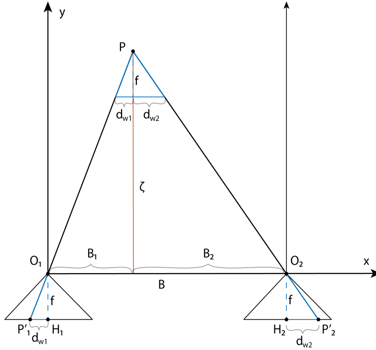
Abbildung 5: Prinzip der Tiefenbestimmung mithilfe von Strahlensätzen für den horizontalen Normalfall. Es zeigt sich, dass die Disparität umgekehrt proportional zur Raumtiefe eines Punktes ist. Je kleiner die Disparität ist, desto größer ist die Entfernung von den Projektionszentren der Kameras. Quelle: [29].
