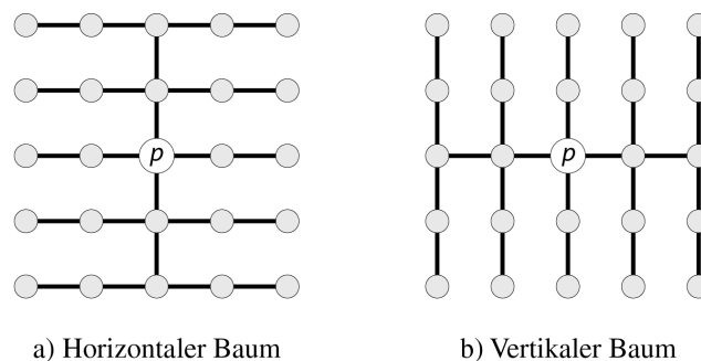
Abbildung 18: Komplementäre Bäume von [9]. Quelle [9].
