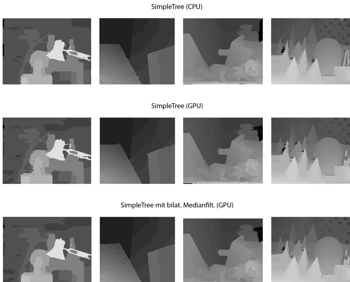
Abbildung 28: Die Ergebnisse der GPU-Implementierung von [9] mit und ohne bilateraler Medianfilterung sowie die Ergebnisse der CPU-Implementierung. Quelle: [9].
