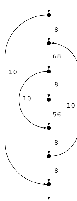
Abbildung 4.2: Beispiel für ein Assemblerprogrammstück und einen entsprechenden T-Graphen
