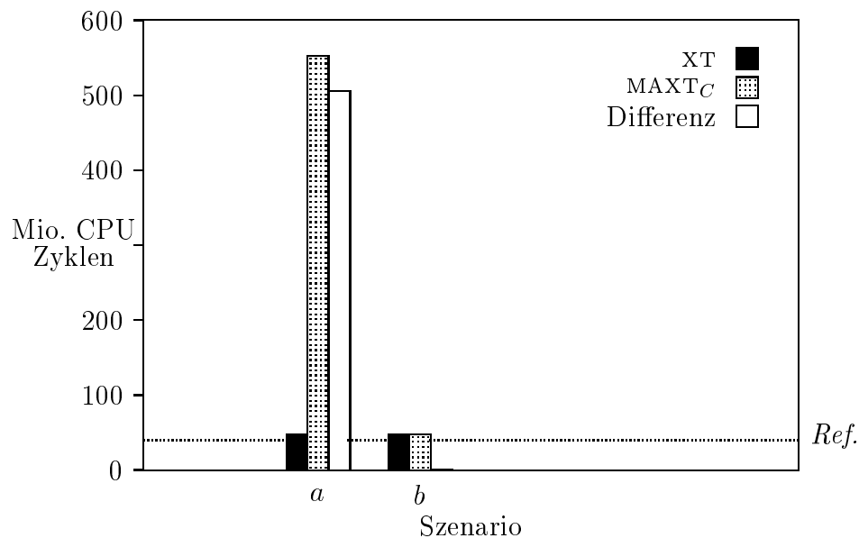
Abbildung 7.12: MAXT und MAXT C von Calculate_Center mit Überprüfung der Restriktionen
