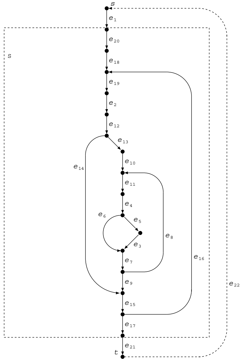
Abbildung A.1: Erweiterter T-Graph für die Bubble Sort Prozedur
