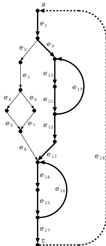
Abbildung 4.5: Eine Zirkulation maximaler Kosten auf einem erweiterten T-Graphen mit Restriktionen.
