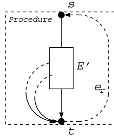
Abbildung 6.4: Erweiterter T-Graph für eine Procedure .
