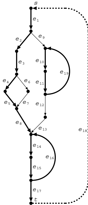
Abbildung 4.4: Eine Zirkulation maximaler Kosten, die keinem gültigen Abarbeitungspfad entspricht. Die fetten Kanten kennzeichnen den zugehörigen Zirkulationssubgraphen.
