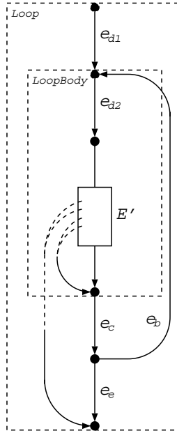
Abbildung 6.8: Graphische Darstellung einer Schleife
