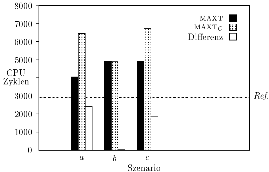
Abbildung 7.10: \text{MAXT} s und \text{MAXT}_C s von Bubble Sort mit Überprüfung der Restriktionen
