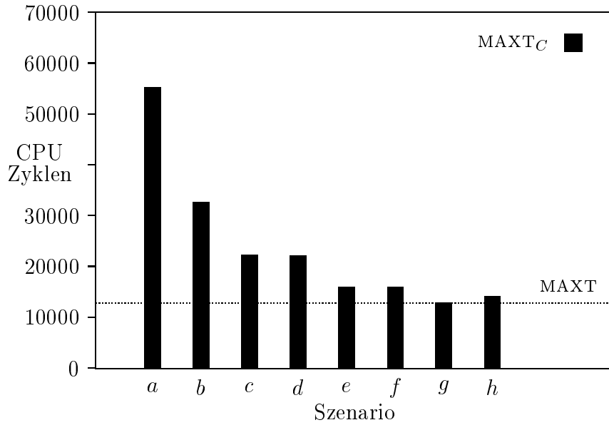
Abbildung 7.7: MAXT C s und MAXT von Sortieren durch Mischen
