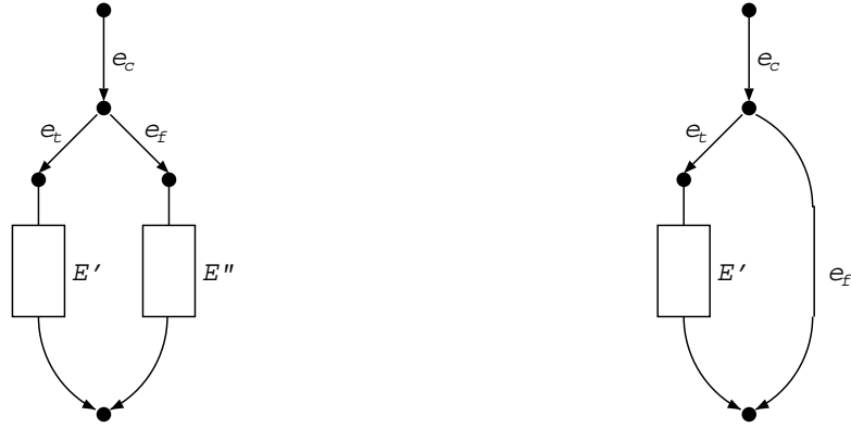
Abbildung 6.7: Graphische Darstellung eines If-Statements mit bzw. ohne Else-Zweig
