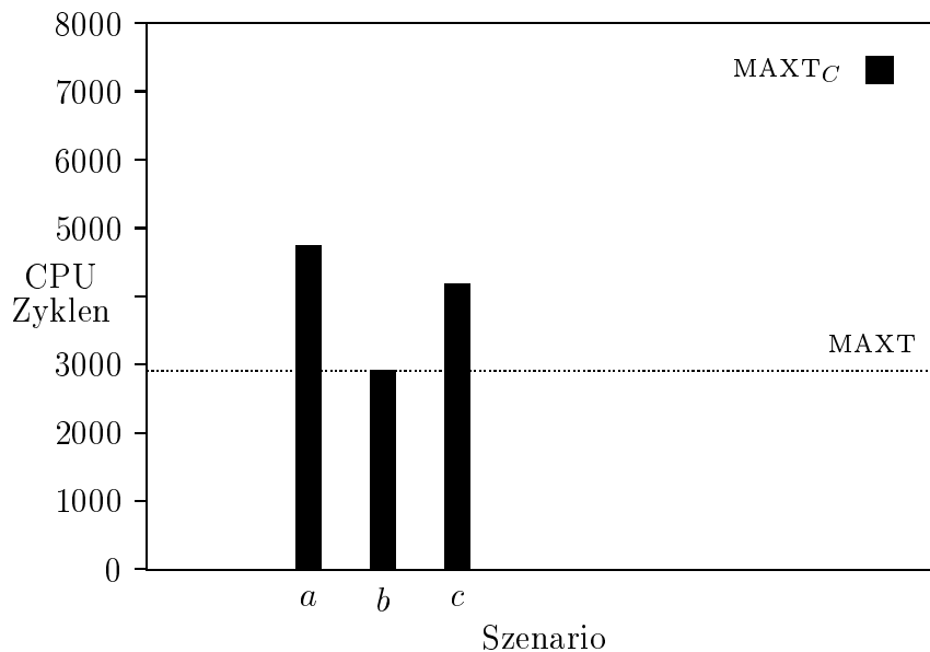
Abbildung 7.6: MAXT C s und MAXT von Bubble Sort
