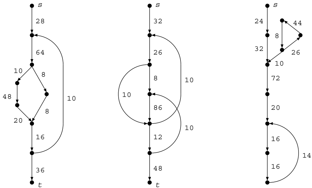
Abbildung 4.1: Zwei gültige T-Graphen (links und in der Mitte) und ein ungültiger T-Graph (rechts), der Eigenschaft 3 verletzt
