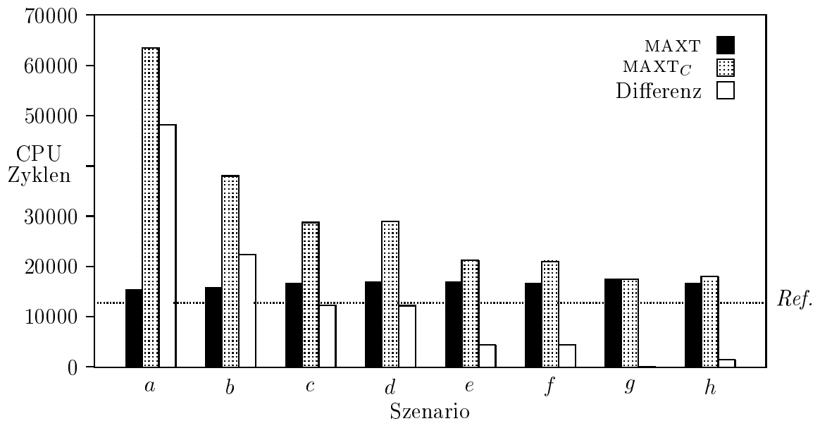
Abbildung 7.11: MAXT und MAXT C für das Sortieren durch Mischen mit Überprüfung der Restriktionen
