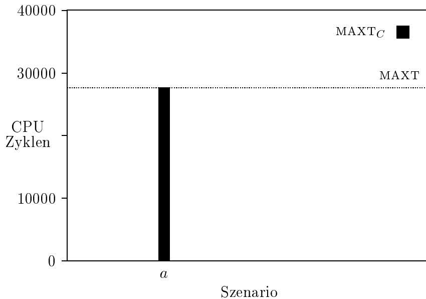
Abbildung 7.5: \text{MAXT}_C und MAXT der Matrixmultiplikation
