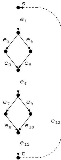
Abbildung 4.6: Ein erweiterter T-Graphen mit Restriktionen, die sich nicht vollständig durch Kapazitätsschranken ausdrücken lassen.
