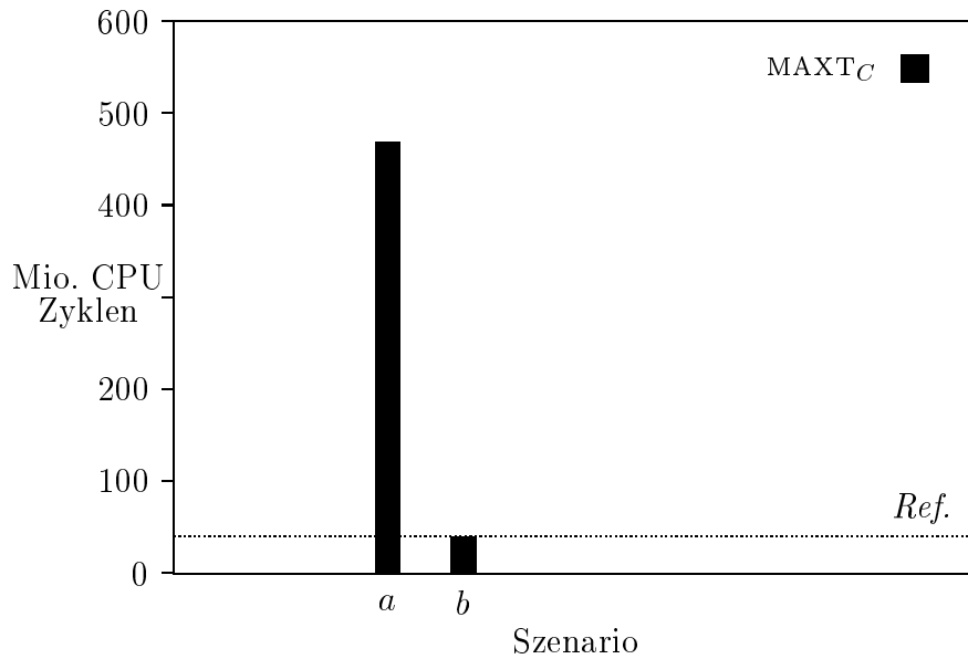
Abbildung 7.8: MAXT C s und Referenzausführungszeit von Calculate_Center
