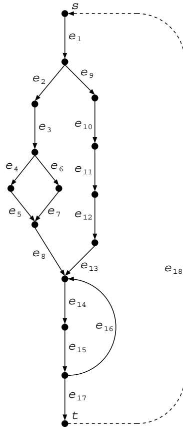
Abbildung 4.3: Beispiel für einen Erweiterten T-Graphen.
