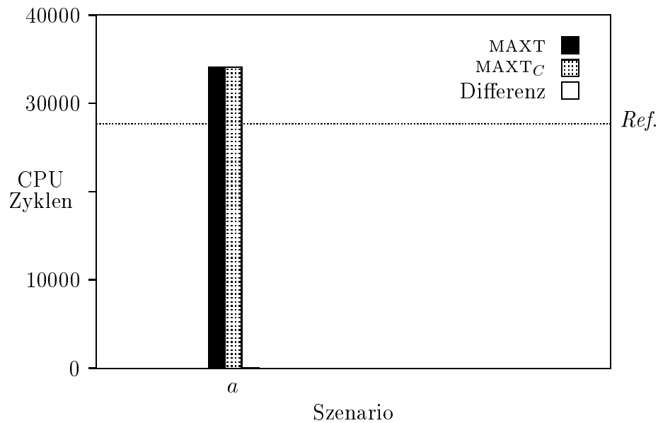
Abbildung 7.9: MAXT und MAXT C der Matrixmultiplikation mit Überprüfung der Restriktionen
