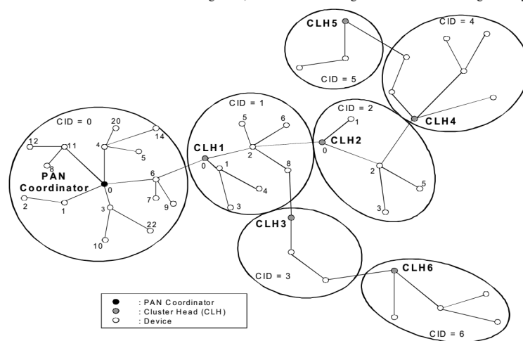
Abbildung 3.17: Aufbau eines Cluster Tree Networks [WPAN03, S.15]
