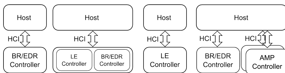
Abbildung 3.4: Mögliche Bluetooth-Konfigurationen
