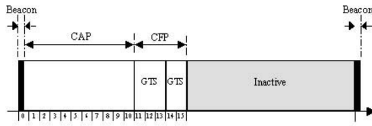
Abbildung 3.18: Aufbau einer Superframe Structure [WPAN03, S.141]
