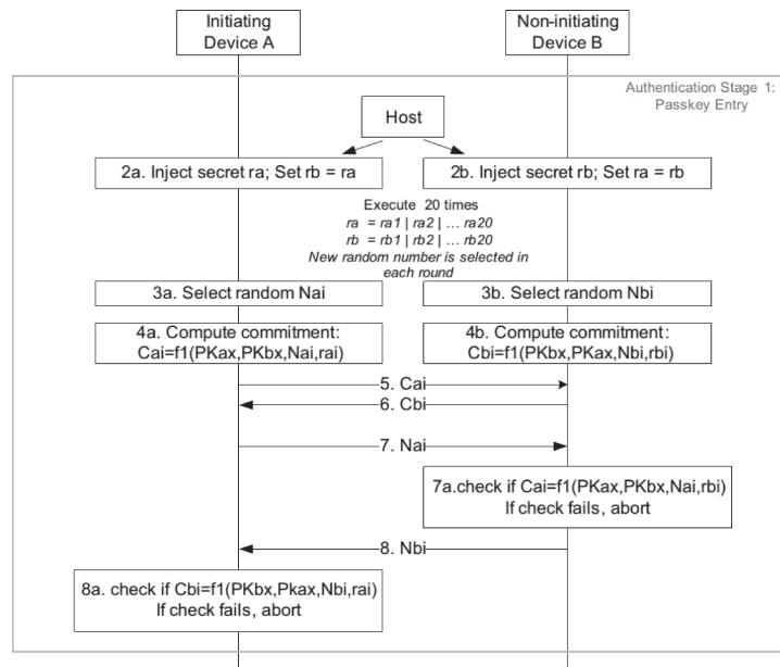
Abbildung 3.10: Passkey Entry Ablaufdiagramm [BLUESTD, S.1656]
