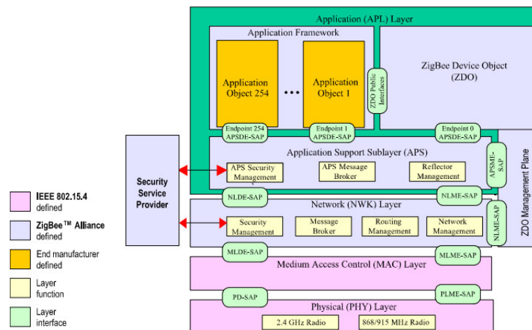
Abbildung 3.16: Schichtenstruktur von ZigBee [ZIGBEESTD, S.2]
