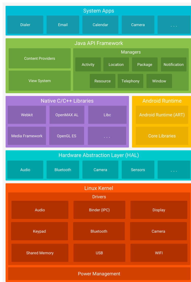
Abbildung 4.5: Architektur von Android ([AND16])
