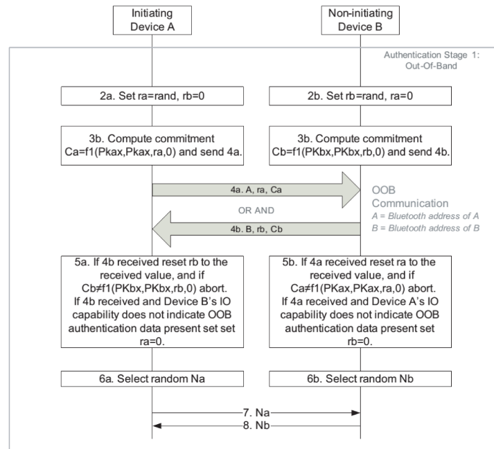
Abbildung 3.11: Out of Band Ablaufdiagramm [BLUESTD, S.1654]
