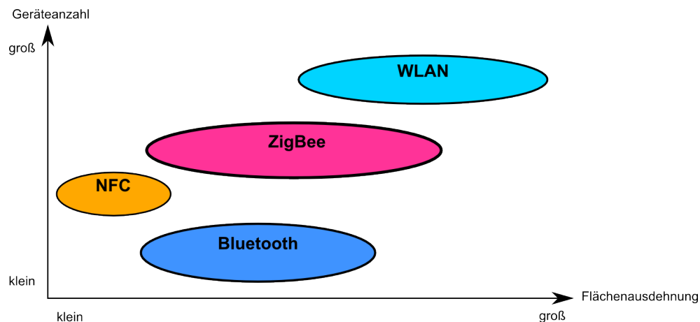
Abbildung 3.19: Vergleich der Protokolle in Bezug auf Anwendungsgebietsgröße und Geräteanzahl
