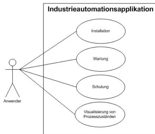
Abbildung 2.1: Use Cases
