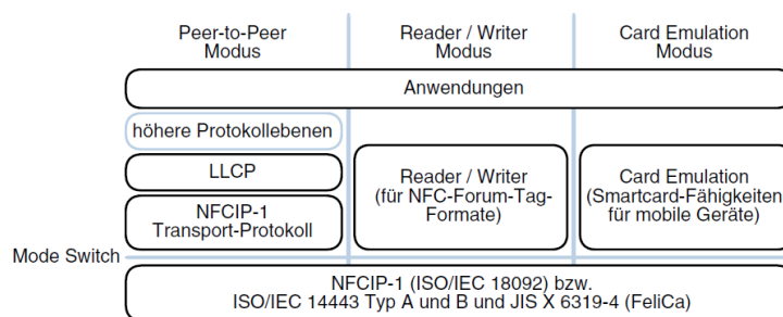
Abbildung 3.13: Aufbau des NFCIP-1 Standards [JLMR10, S.90]
