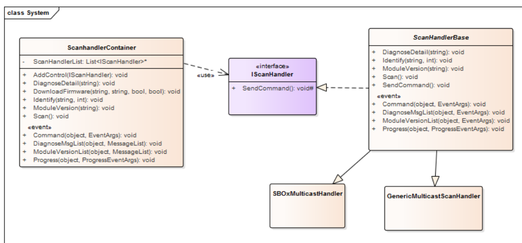
Abbildung 5.2: Vereinfachtes Klassendiagramm des Systems
