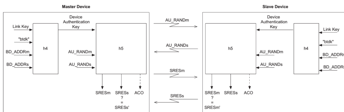
Abbildung 3.12: Authentifizierung Ablaufdiagramm [BLUESTD, S.1640]
