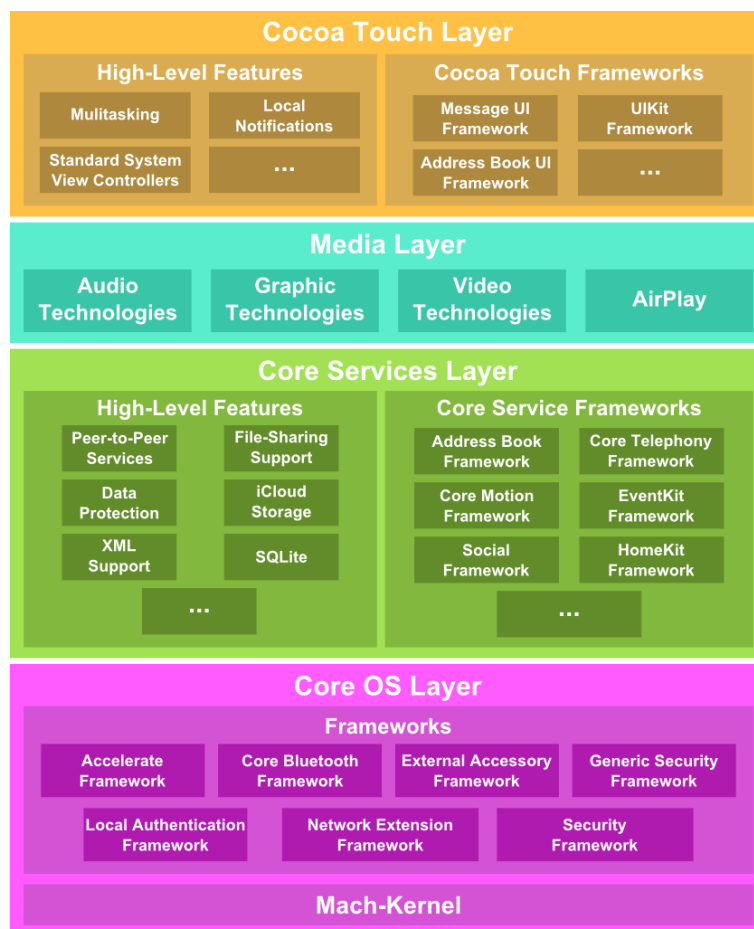
Abbildung 4.6: Aufbau von iOS
