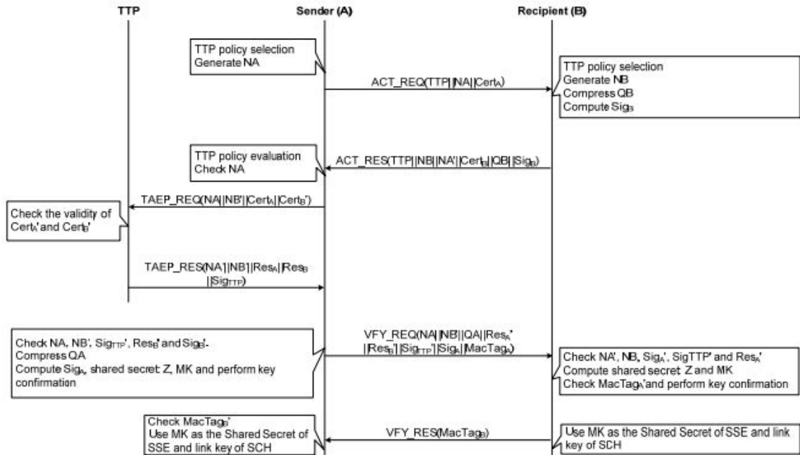
Abbildung 3.15: Asymmetrische Schlüsselgenerierung [NFCIP-5, S.13]
