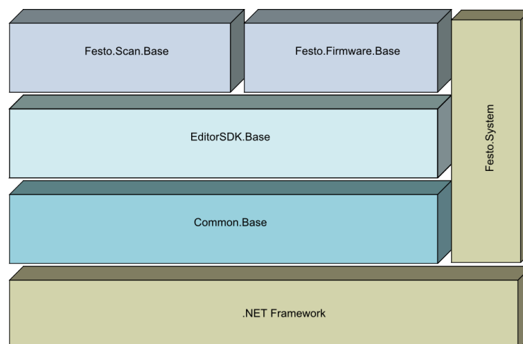
Abbildung 5.1: Schichtenaufbau der Anwendung
