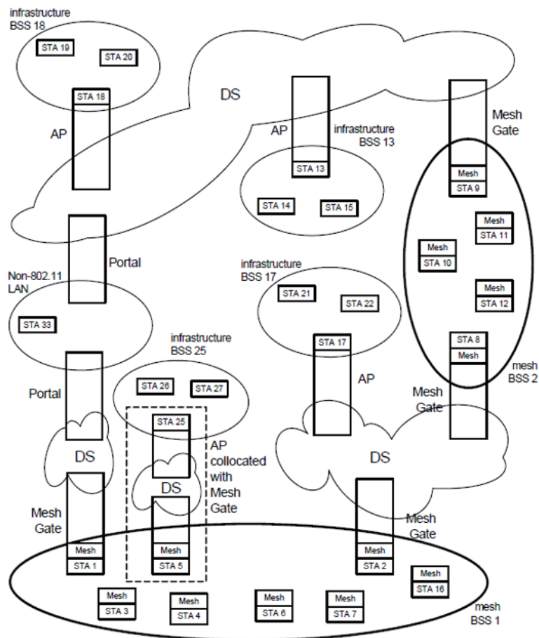
Abbildung 3.3: Mesh BSS Beispielkonfiguration [IEEE2, S.63]
