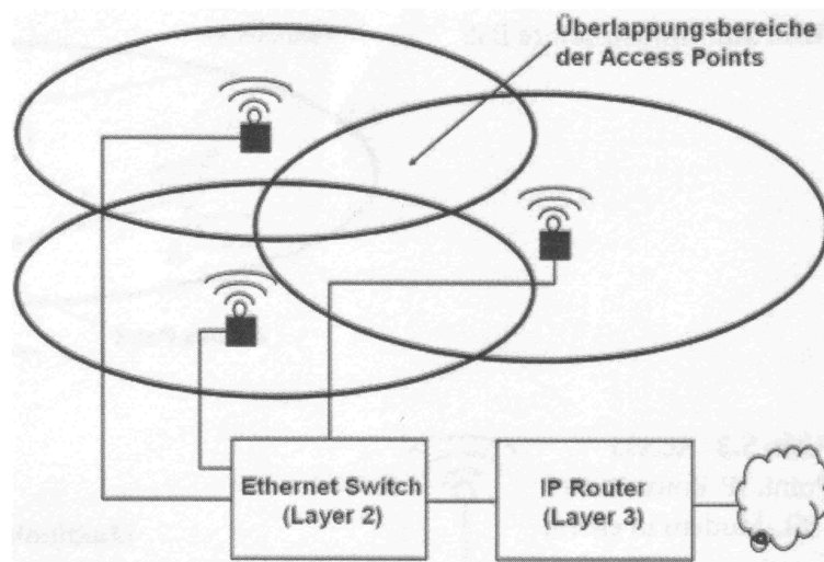
Abbildung 3.2: ESS Schema [PROT2012, S.302]
