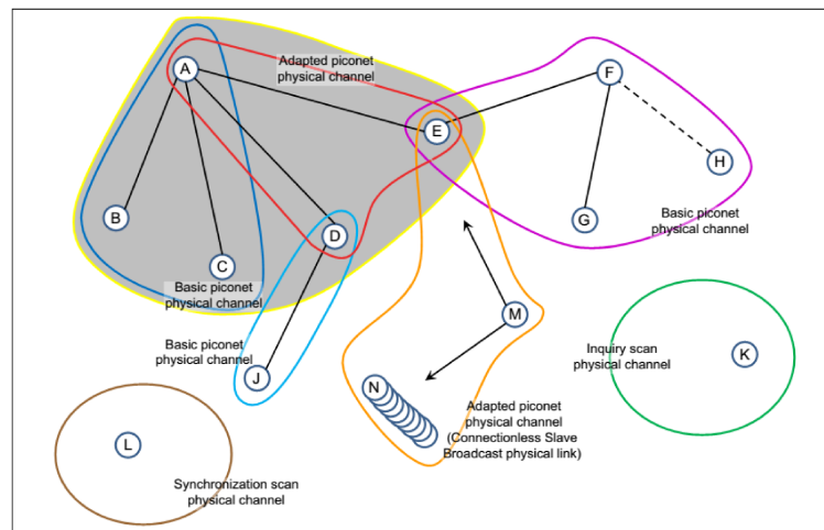
Abbildung 3.6: Pico-Netz Konfigurationen [BLUESTD, S.228]
