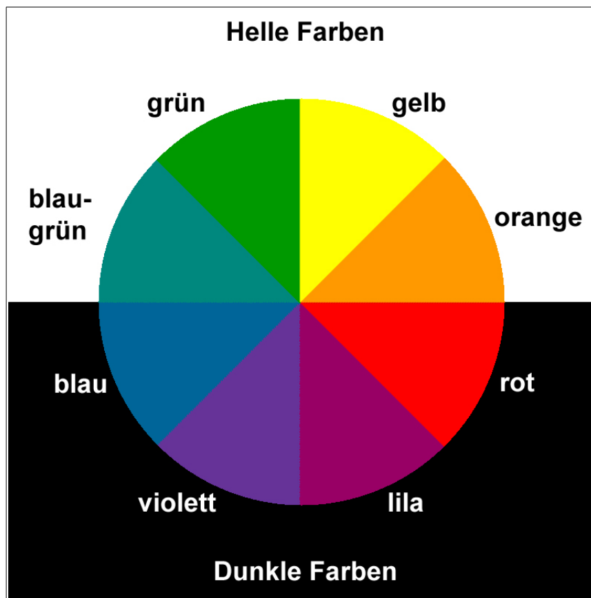
Abbildung 5.11.: Farbspektrum.
